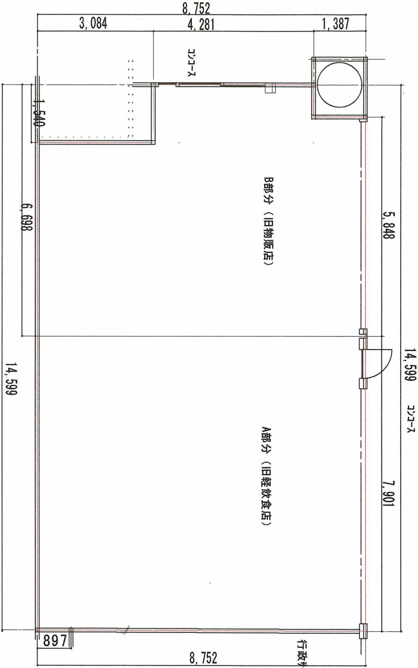
平面図 S=1/100
