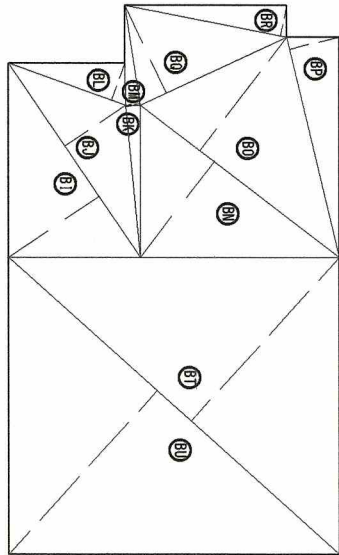
求積図 S=1/200
